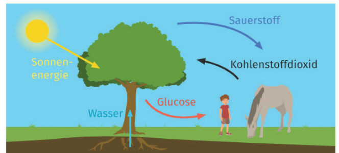
Der CO 2 -Kreislauf – Voraussetzung für das Leben auf der Erde
